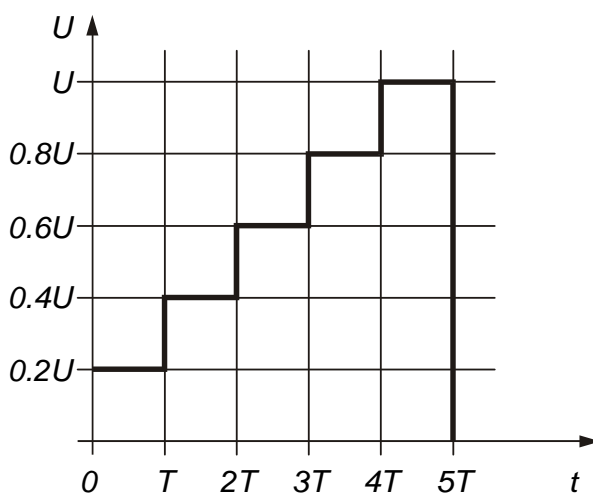
Fig. 24. Step-up test voltage
